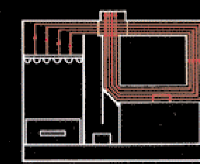
Percorso fumi minimo riscaldamento e massimo forno cottura in una CTF.
