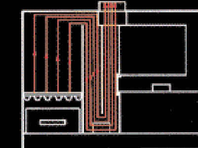
Percorso fumi massimo riscaldamento e minimo forno cottura in una CTF.
